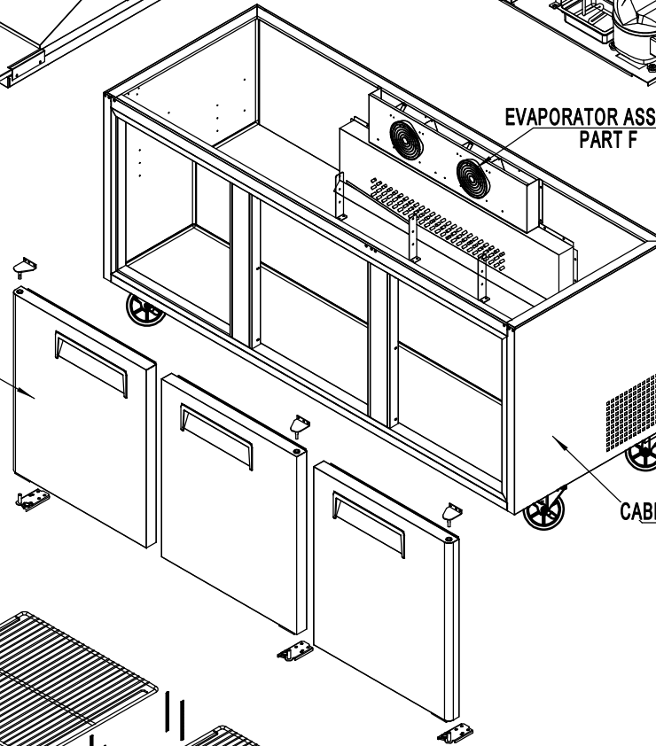
DOOR ASSEMBLY PART B
